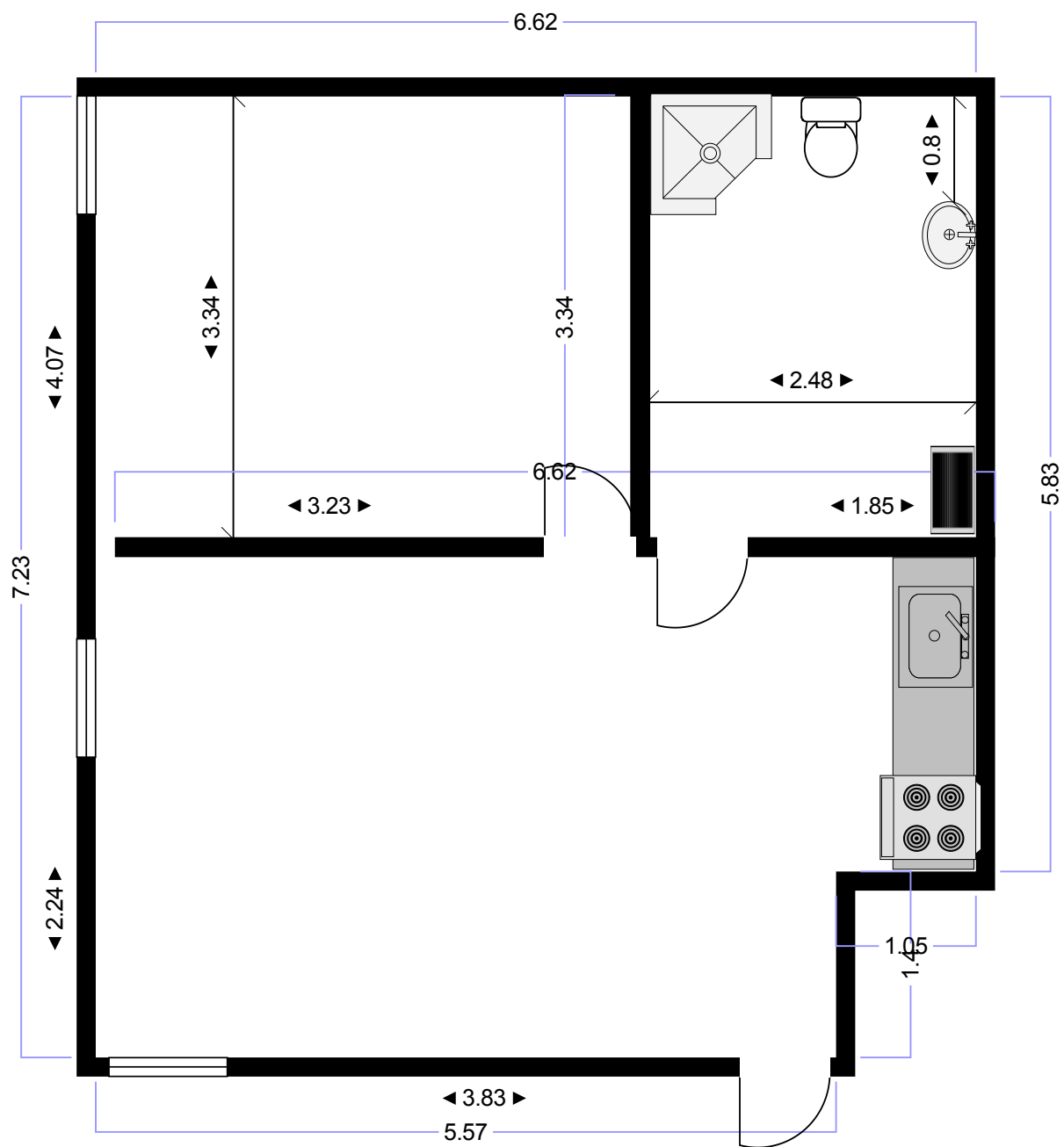
appartement Stationsstraat 65 Beganegrond C2 ongeveer 46m2
