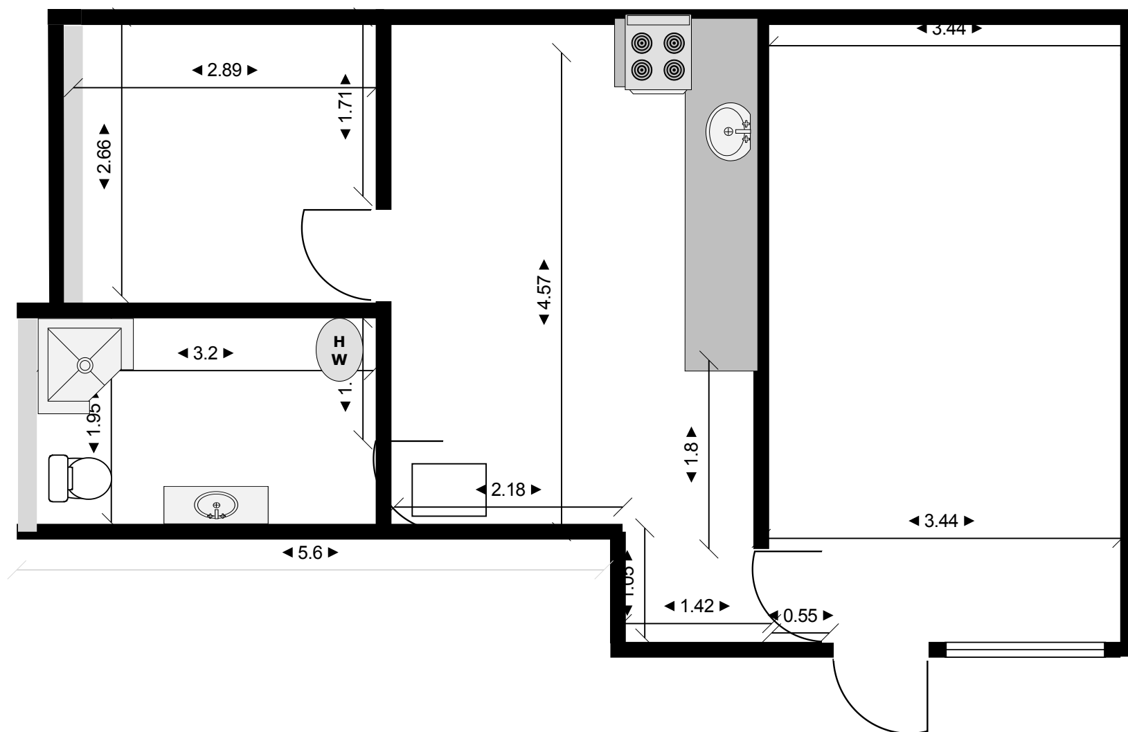
Appartement Stationsstraat 65 Begane grond C3 50m2
